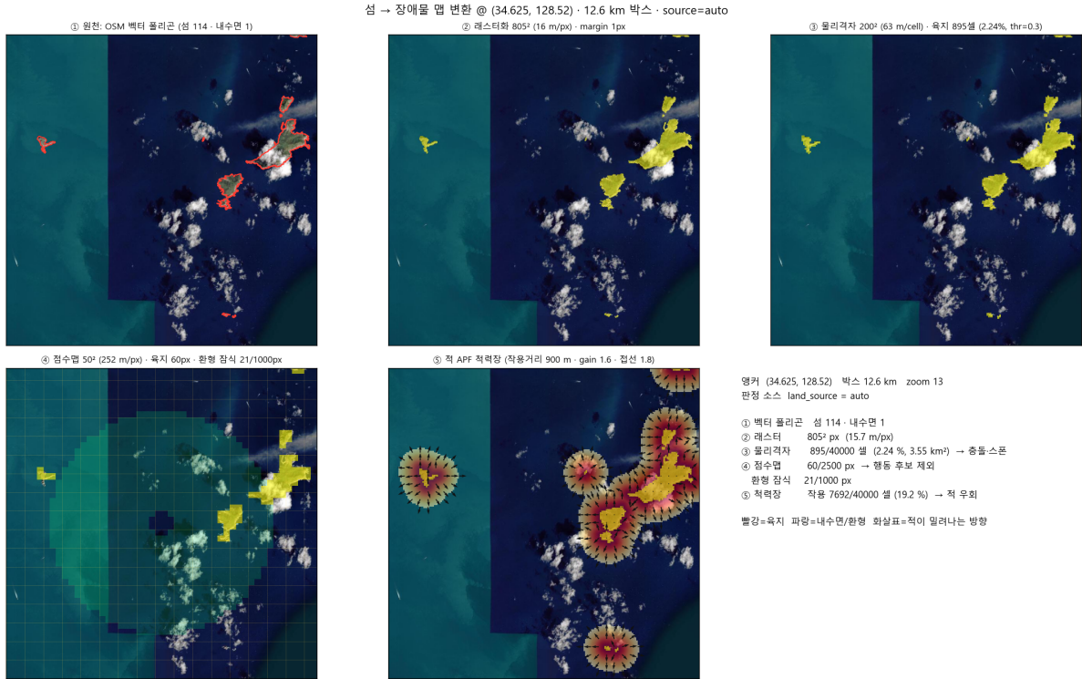
Figure 5: 실해역 지형의 반영 과정(통영 매물도 인근, 12.6 km 박스). ① OpenStreetMap 벡터 폴리곤 → ② 고해상도 래스터 (805 2 , 16 m/px) → ③ 충돌 판정용 물리 격자(200 2 , 63 m/cell) → ④ 정책 격자(50 2 , 252 m/px)로 면적비 다운샘플. 판정과 관측을 다른 해상도로 두는 이유는 충돌은 이진 판정을 요구하고, 관측은 해안선이 계단으로 들어가면 안 되기 때문이다. ⑤는 적의 우회를 유도하는 적력장으로, 관측이 아니라 적 기동 모형의 일부다.
