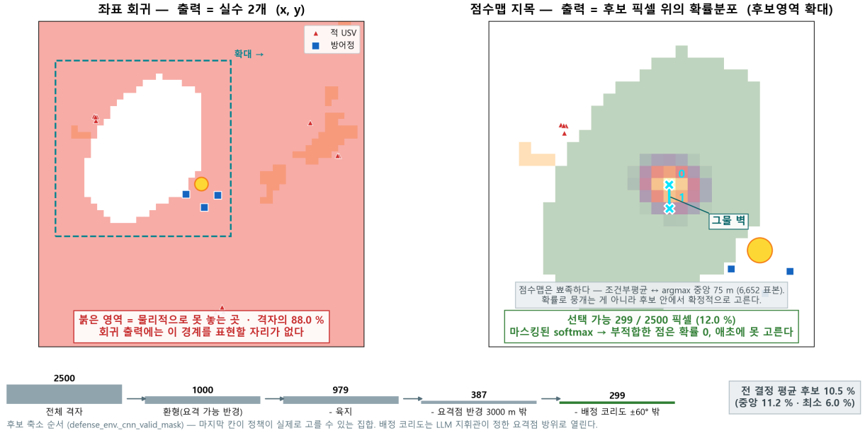
Figure 7: 왜 좌표 회귀가 아니라 점수맵 위 픽셀 지목인가(학습된 체크포인트의 실제 출력). 왼쪽: 연속 좌표를 회귀하는 출력에는 “놓을 수 없는 곳”을 표현할 자리가 없다 — 이 장면에서 붉은 영역이 격자의 88.0%다. 오른쪽: 같은 장면을 후보 영역으로 확대한 점수 분포와 선택된 두 픽셀, 그리고 그 둘을 잇는 그물벽이다. 마스크된 softmax 아래에서 부적합한 칸은 확률이 0이라 애초에 선택되지 않는다. 아래 막대 는 제약이 순차 적용되며 후보가 줄어드는 과정이다 (2500 → 1000 → 979 → 387 → 299, 12.0%). 전 결정 평균 후보는 10.5%였다.
