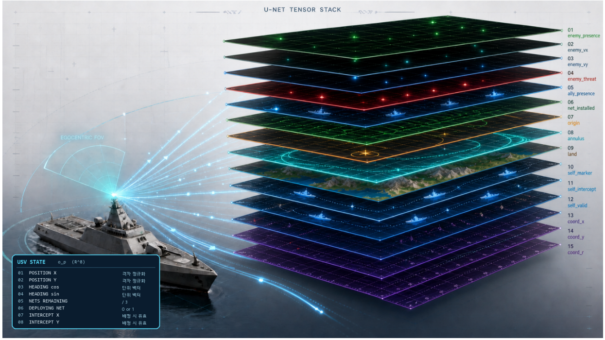
Figure 4: 15채널 관측의 구성. 전역 9채널(01-09), 방어정별 3채널(10-12), 좌표 3채널(13-15)이 같은 50 \times 50 격자에 겹쳐 하나의 다채널 영상을 이룬다. 오른쪽의 채널 이름은 구현의 이름과 같다. 왼쪽 아래는 격자에 담기지 않고 벡터로 들어가는 방어정 자체 상태 \mathbf{o}_p \in \mathbb{R}^8 — 위치 2, 헤딩 단위벡터 2, 잔여 그물 1, 전개 중 여부 1, 배정 요격점 2이며, 요격점 두 성분은 배정이 없으면 0이다. 그림의 좌측 시선원뿔(“egocentric FOV”)과 함정 형상은 삽화의 표현이다 — 본 연구의 래스터는 방어정 시야가 아니라 모션을 중앙에 둔 전역 격자이며, 방어정마다 달라지는 것은 3채널(10-12)과 \mathbf{o}_p 뿐이다.
