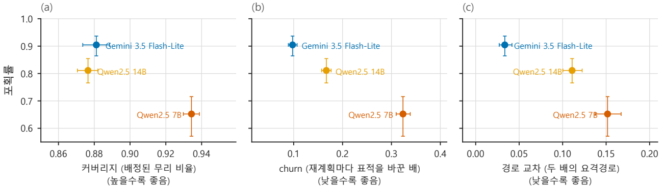
Figure 14: 계획 품질(가로축)과 성능(세로축). 점 하나가 지휘관 모델 하나이고 오차막대는 양방향 부트스트랩 95% 신뢰구간이다. 세 패널의 대조가 핵심이다 — (a) 커버리지는 성능과 같이 움직이지 않는다(7B가 커버리지 최고, 성능 최저). (b) churn과 (c) 경로 교차는 성능과 단조로 반대 방향이다. 회귀선이나 상관계수는 없지 않았다. 모델이 3종이라 n = 3 이며, 여기에 상관을 적으면 없는 통계적 근거를 주장하는 셈이 된다.
