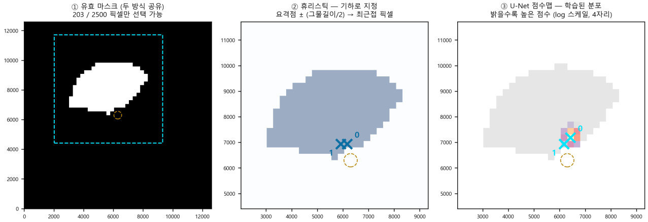
Figure 3: 기동 계층 두 방식의 비교(학습된 체크포인트의 실제 출력, 같은 전장·같은 시점). 왼쪽: 두 방식이 공유하는 유효 마스크 — 2500칸 중 203칸만 선택 가능하다. 가운데: 휴리스틱은 유효 영역 안에서 기하로 정해진 두 점을 지목하며, 나머지 칸에 대한 선택을 표현하지 않는다(영역 전체가 균일하게 칠해져 있다). 오른쪽: 점수맵 정책은 같은 영역 위에 학습된 분포를 얹어 소수의 칸에 확률을 집중시킨다. 두 방식은 같은 격자·같은 마스크·같은 거리 제약을 통과한다 — 행동공간이 동일해야 성능 차이가 방법의 차이가 된다.
