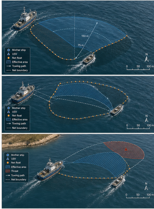
Figure 16: 실제 그물 전개가 갖는 형상(참고). 두 척이 그물을 예인하면 벽이 아니라 곡선으로 펼쳐진 면적이 만들어지고, 그 면적이 위협 방향과 얼마나 겹치는지가 차단 성능을 좌우한다. 본 연구의 모형은 이를 단순화하여, 방어정 한 척이 두 좌표를 잇는 직선 그물벽을 치고 그 선분에 적선이 닿으면 포획되는 것으로 처리한다. 전개 곡률, 예인 편대, 면적의 시간 변화는 반영하지 않는다. 그림의 치수 또한 개념 전달을 위한 것으로 본 연구의 설정(최대 450m)과 다르다.
