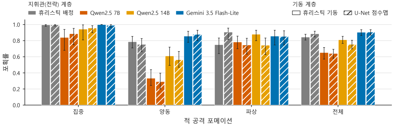
Figure 10: 포메이션 × 조건 포획률. 색은 전략 계층(지휘관), 빗금은 기동 계층을 나타내며, 같은 색 안에서 인접한 두 막대가 곧 그 지휘관에서의 U-Net 효과이다. 무채색 두 막대는 언어모델을 쓰지 않는 기준선이고, 그 오른쪽부터가 언어모델 지휘관이며 모델 규모 오름차순으로 놓았다 — 성능 순서가 아니다. 실제로 7B는 기준선보다 낮다($6.6). 오차막대는 표준편차가 아니라 시드 부트스트랩 95% 신뢰구간이다. 집중 포메이션에서 여덟 조건이 모두 상단에 몰려 있는 것이 천장 효과이며($6.3), 양동 포메이션에서만 지휘관 능력축이 넓게 벌어진다.
