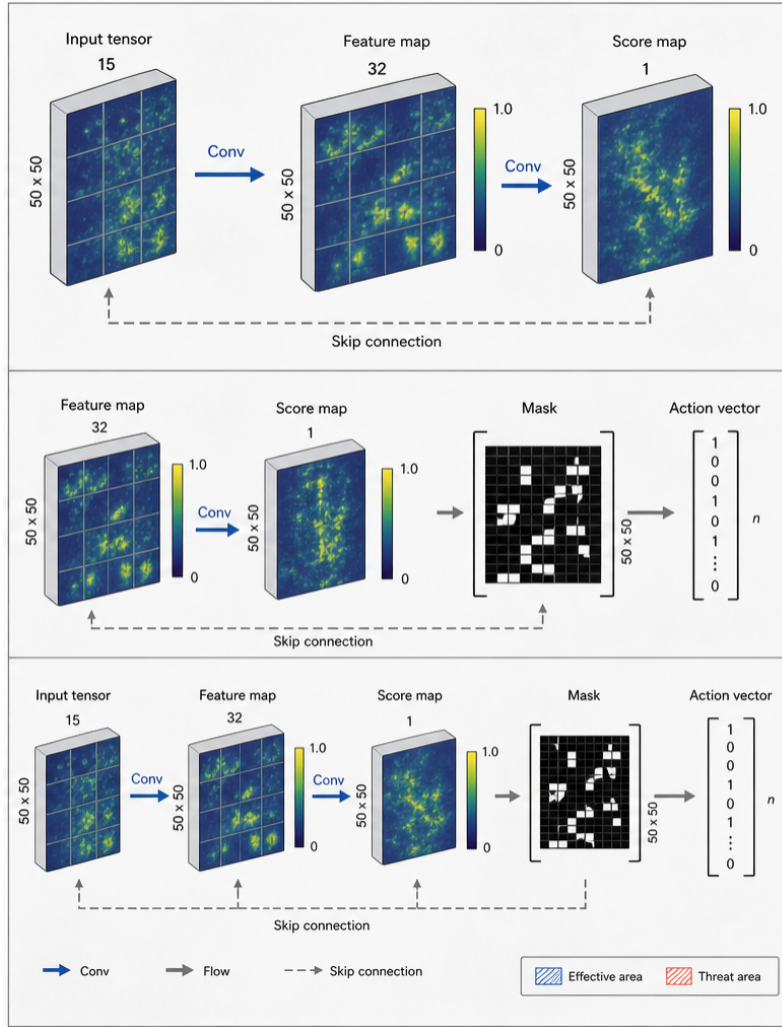
Figure 17: 기동 계층의 텐서 흐름. 15채널 입력( 50 \times 50 )이 합성곱을 거쳐 32채널 특징 지도가 되고, 다시 1채널 점수맵이 된다. 유효 마스크가 점수맵에 곱해져 선택 가능한 칸만 남기고, 그 위에서 지목한 픽셀이 행동 벡터가 된다. skip 연결이 입력과 특징 지도의 위치 정보를 점수맵으로 전달한다. 세 행은 같은 흐름을 단계별로 나누어 보인 것이다.
