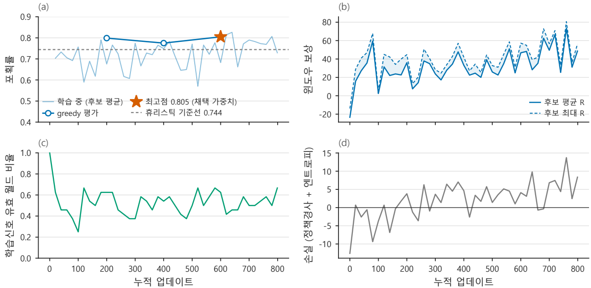
Figure 8: GRPO 학습 경과( 50^2 격자, 후보 G = 8 , 후보 평가 구간 180step, 실패역 6곳 로테이션, 800 업데이트). (a) 포획률. 열은 선은 학습 중 후보 평균, 원 표식은 200 업데이트마다의 greedy 평가, 회색 파선은 휴리스틱 기준선 0.744이다. 별표(600 업데이트, 0.805)가 본 논문이 평가하는 가중치이다. (b) 후보 평균 보상과 후보 최대 보상 — 둘의 간격이 그룹 내 변별력이다. (c) 후보 간 분산이 0이 아닌 월드의 비율(학습 신호가 실제로 생긴 비율). (d) 손실(정책경사 + 엔트로피). 부호와 크기 자체는 수렴 지표가 아니다.
