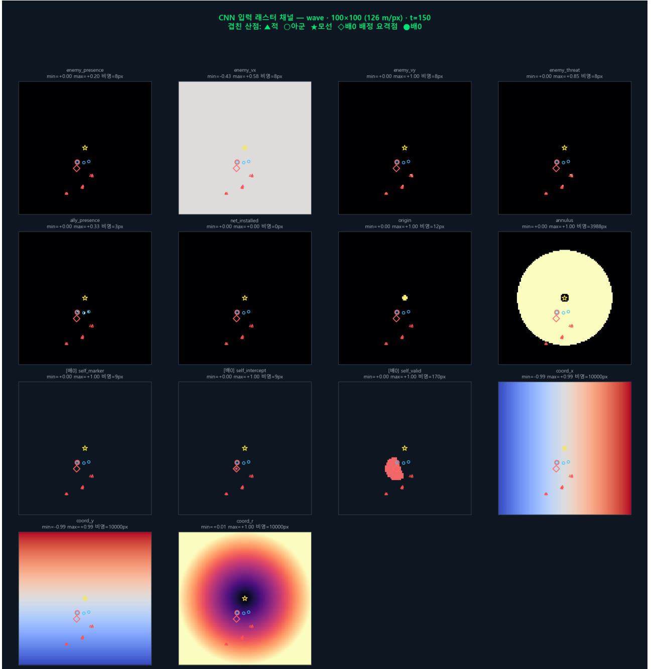
Figure 18: 래스터화된 다채널 관측의 채널별 분해. 전역 채널(적 밀도, 적 진행 x \cdot y , 적 위협도, 아군 위치, 설치된 그물, 원점, 요격 환경), 방어정별 채널(자기 위치, 배정 요격점, 유효 영역), 좌표 채널( x, y, r )이 같은 격자에 정렬된다. 각 패널에 min/max 와 비영 픽셀 수를 함께 표시하였다. 이 그림은 시각적 판독을 위해 100 \times 100 (126 m/px)로 렌더하였다 — 본문의 학습·평가 설정은 50 \times 50 (252 m/px)이며 채널 구성과 의미는 동일하다. 육지 채널은 이 장면에 육지가 없어 표시되지 않았다.
