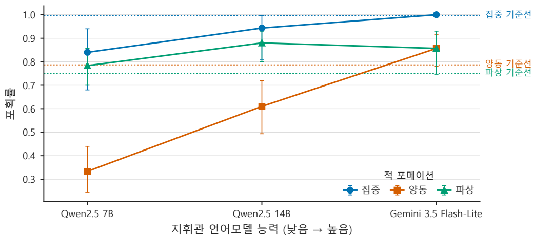
Figure 13: 지휘관 능력 사다리(기동 계층은 휴리스틱으로 고정). 점선과 오른쪽 이름표는 같은 포메이션의 휴리스틱 배경 기준선이고, 오차막대는 시드 부트스트랩 95% 신뢰구간이다. 판건은 성능이 오르는지가 아니라 어디에서 기준선을 교차하는 가이다 — 양동 포메이션에서 7B와 14B는 기준선 아래에 있고 Gemini에서 처음 위로 올라선다. 집중 포메이션은 기준선이 0.997로 천장이지만 세 모델이 거기 붙어 있는 것은 아니다 — Gemini만 기준선에 닿고, 7B는 0.840으로 기준선보다 유의하게 낮다. 천장은 개선 여지를 없앨 뿐 악화 여지를 없애지 않는다($6.3).
